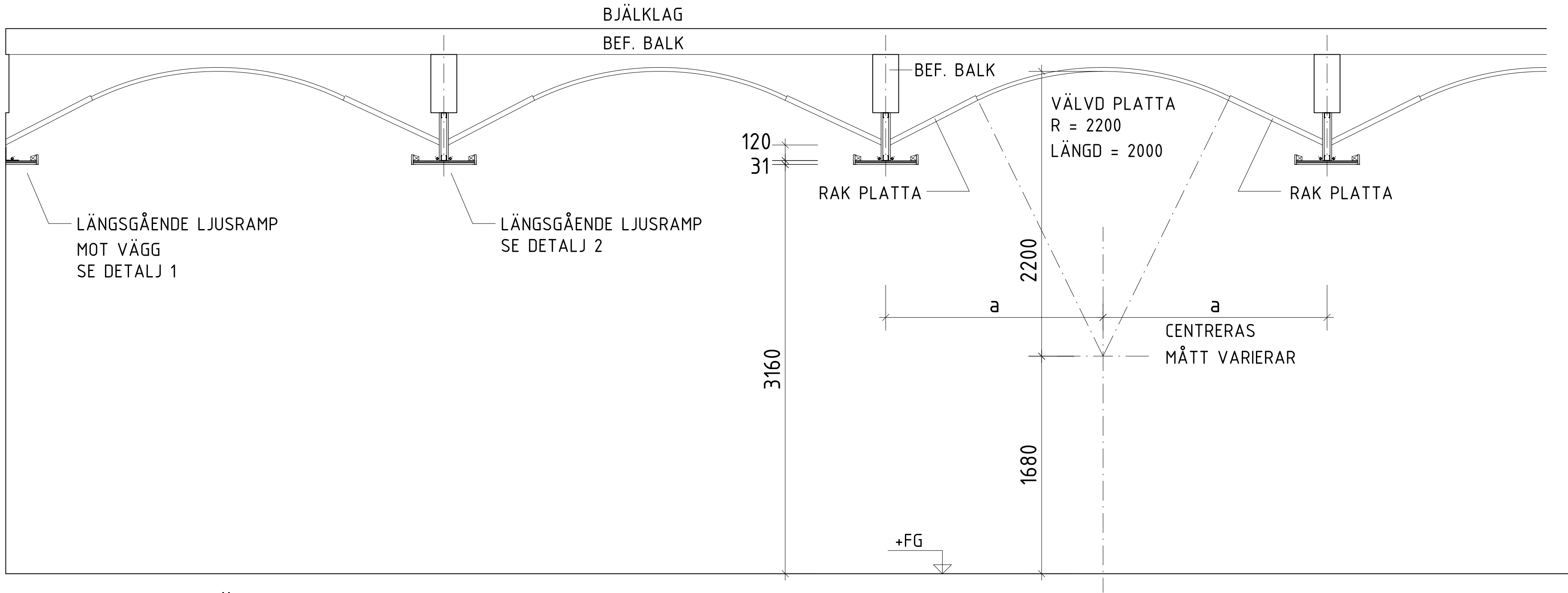
PRINCIPSEKTION VÄLVD UNDERTAK SKALA 1:25
