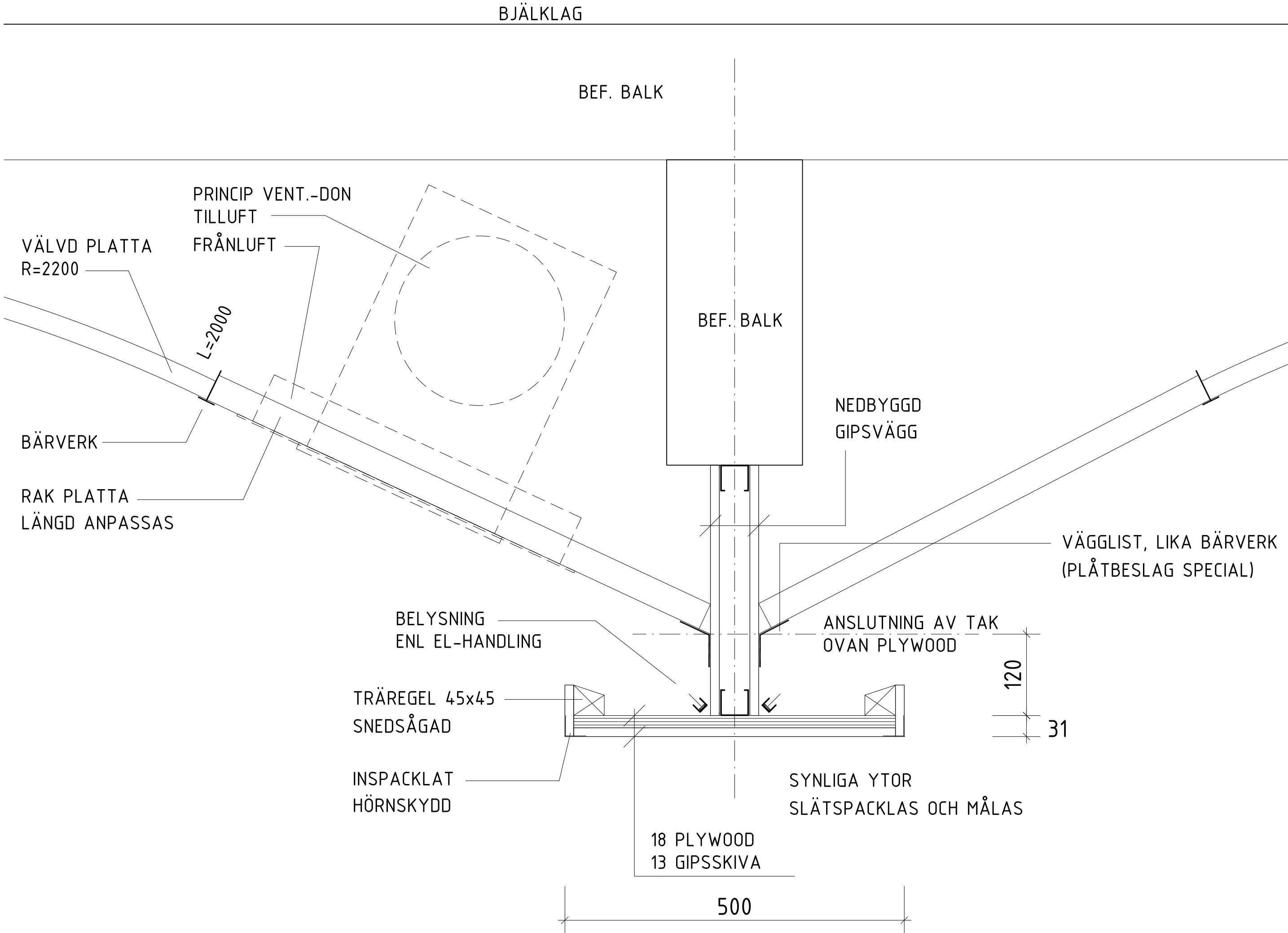
DET. 2 LÄNGSGÅENDE LJUSRAMP SKALA 1:5
